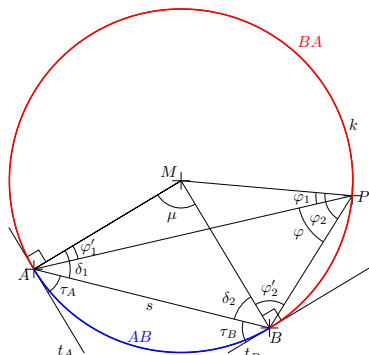
Illustration 2.16.9 der Kreiswinkelsätze
